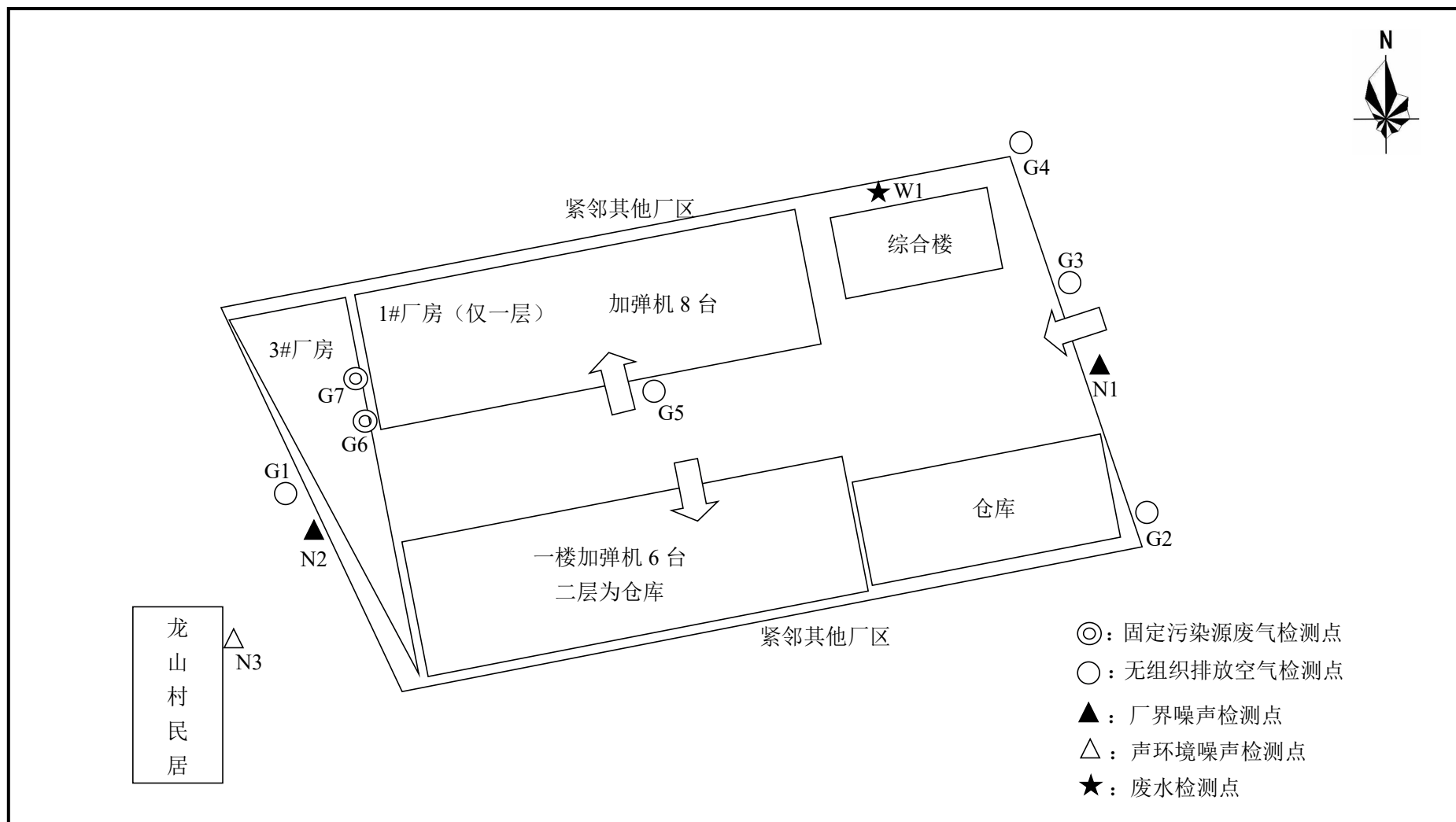
图 7-1 本项目监测点位图
