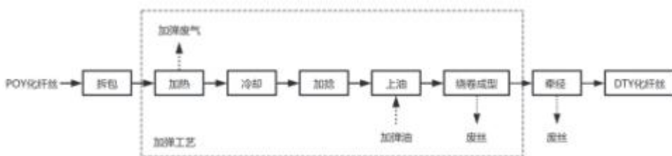
图 3-4 本项目化纤丝生产工艺及产污流程图
