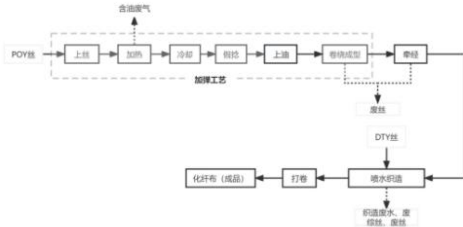
图 3-4 本项目高端纺织面料生产工艺及产污流程图
