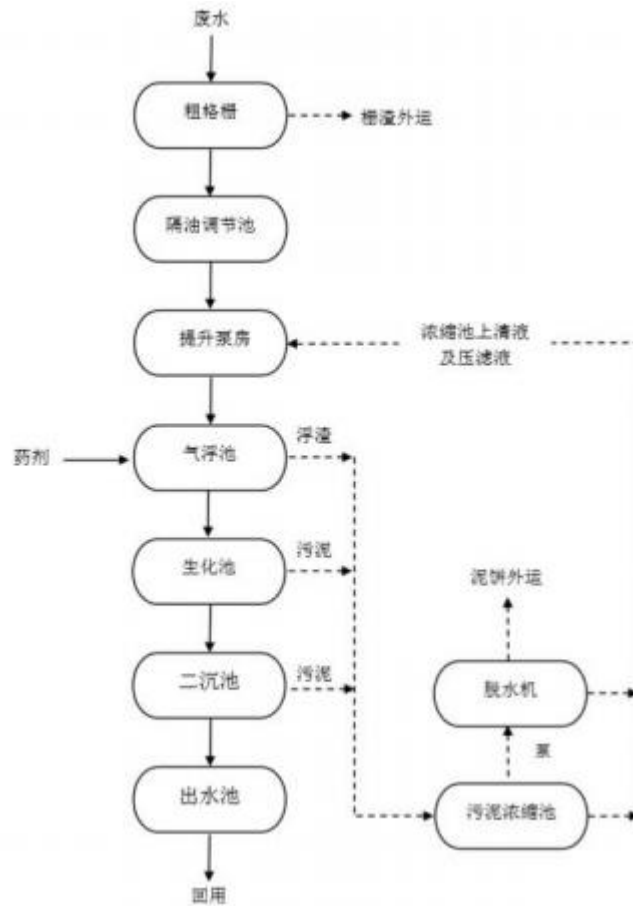
图 4-1 本项目织造废水中水回用站处理工艺流程图
