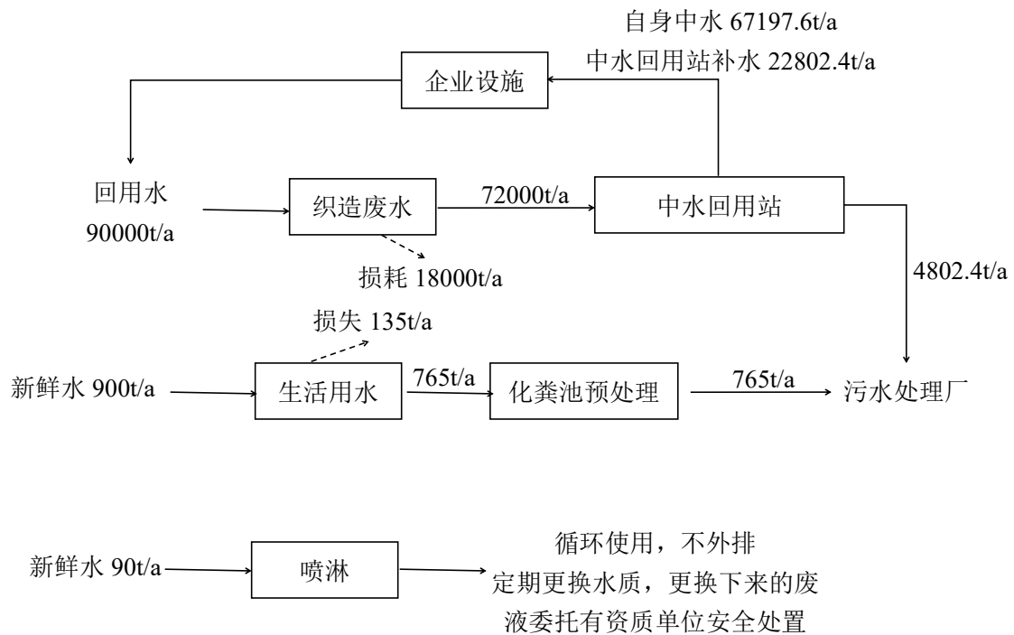
图 3-4 本项目水平衡图
