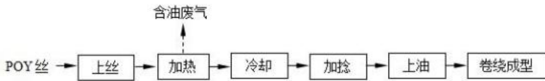
图 3-6 加弹工艺及产污流程图
