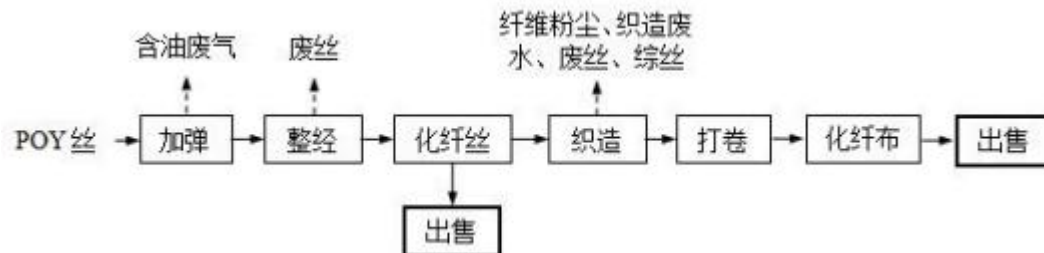
图 3-5 化纤布、化纤丝生产工艺及产污流程图
