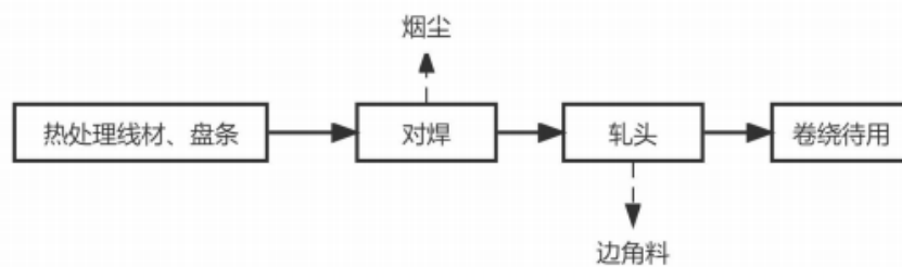
图 3-5 本项目预处理生产工艺及产污流程图
