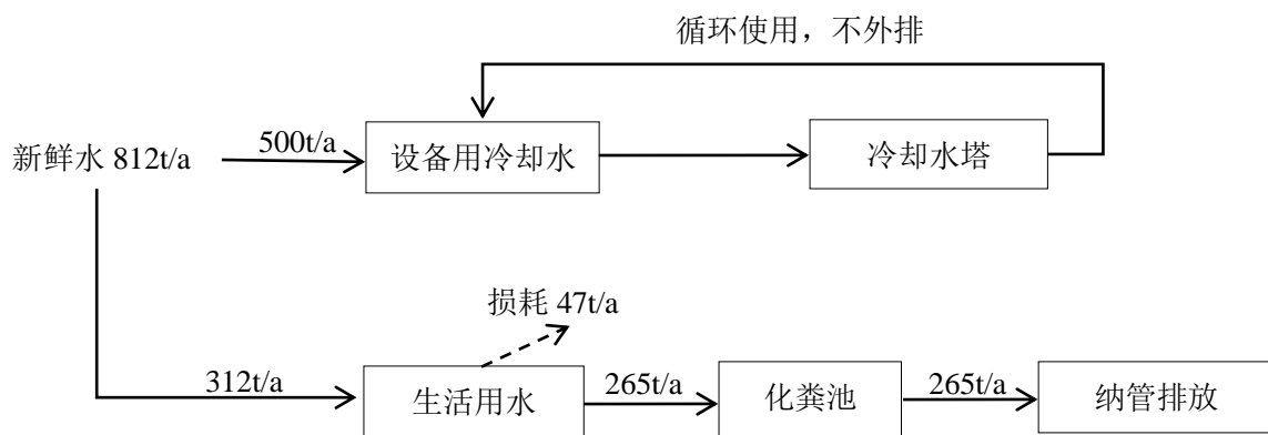
图 3-4 本项目水平衡图
