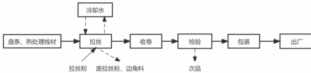
图 3-6 本项目光缆用钢丝、钢琴丝、弹簧钢丝生产工艺及产污流程图
