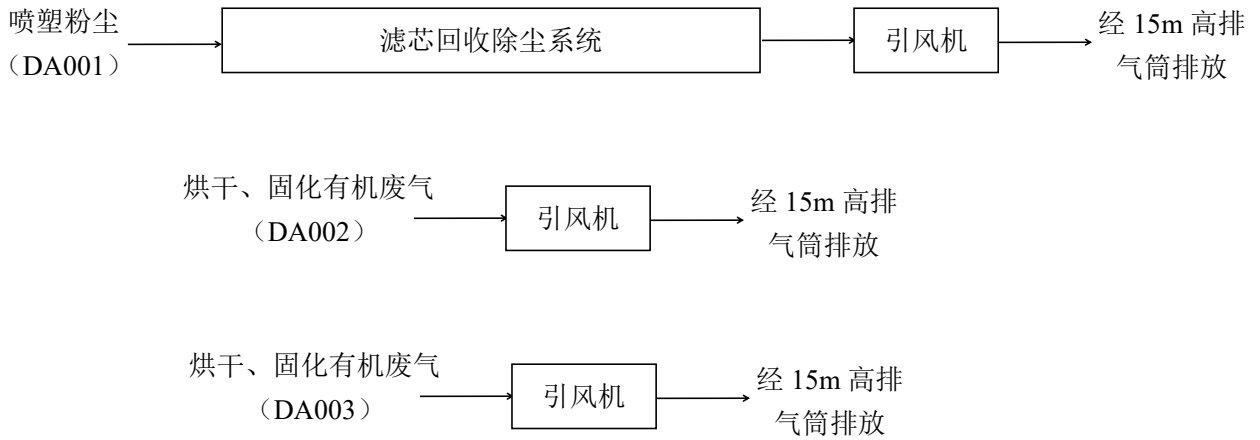
图 4-2 项目废气处理工艺流程图
