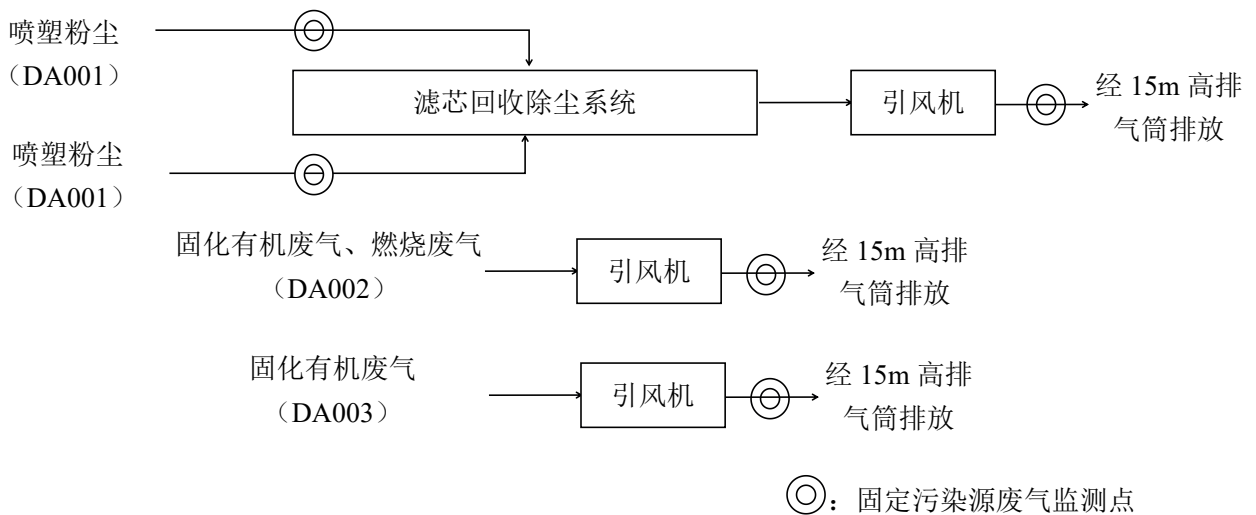
图 7-1-1 项目废气处理工艺流程及废气监测点位示意图
