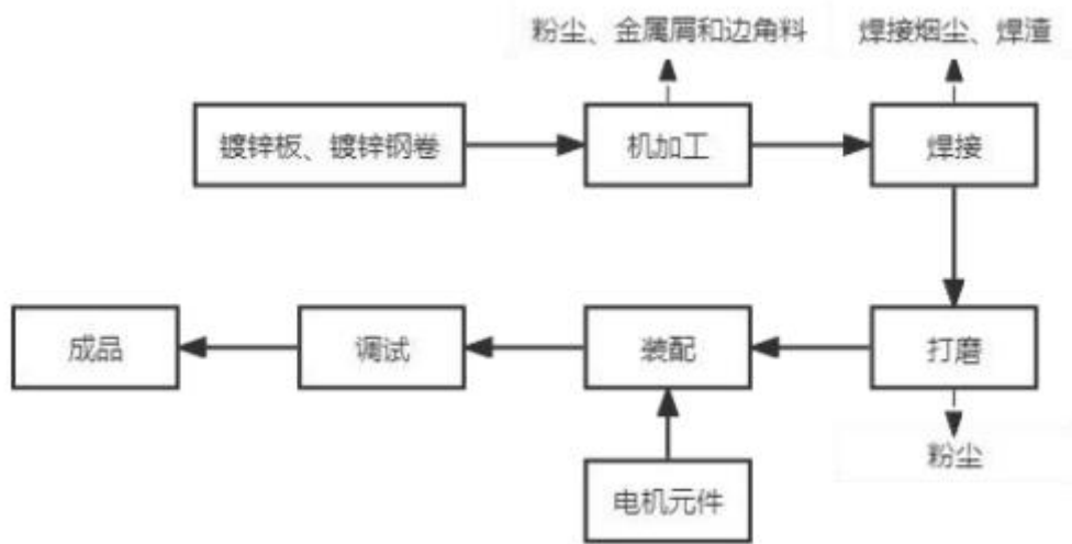
图 3-5 本项目镀锌桥架生产工艺流程及产污环节示意图
