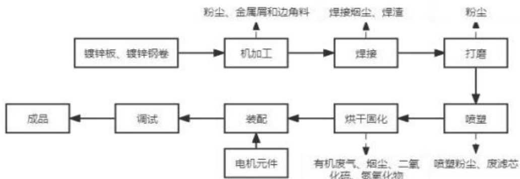
图 3-4 本项目防火桥架、喷塑桥架生产工艺流程及产污环节示意图
