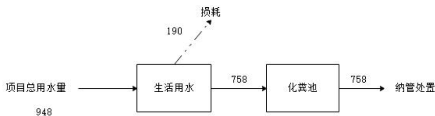
图 3-4 项目水平衡图 (单位: t/a)
